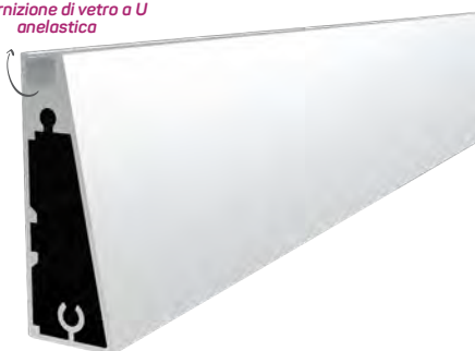
Guarnizione di vetro a U anelastica
